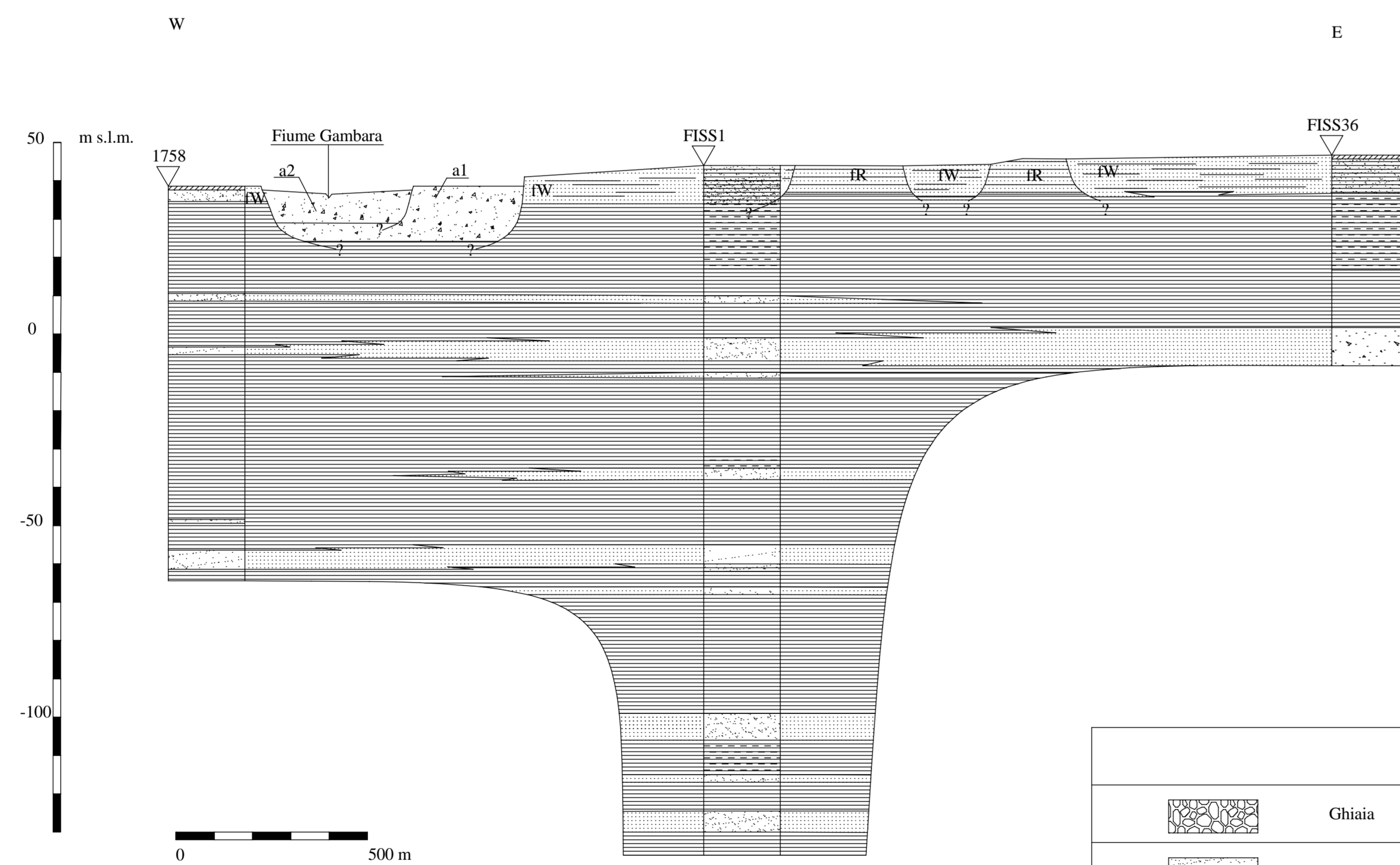
SEZIONE 2
