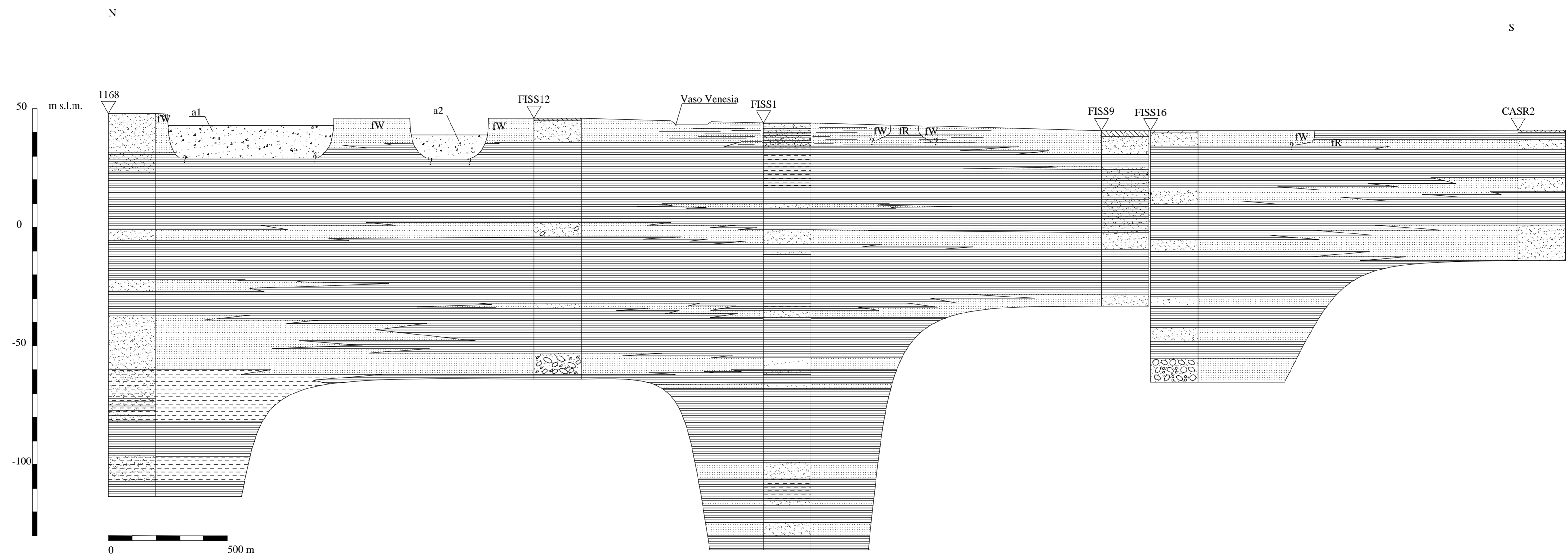
SEZIONE 1
